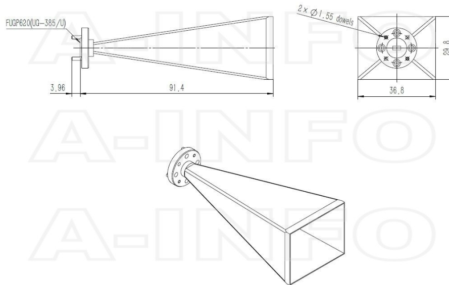
FUGP620 Output (P/N: LB-15-25-A)
